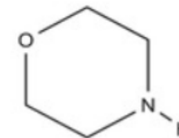
D: Morpholine
